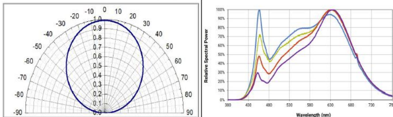
Viewing Angle Distribution 发光角度
